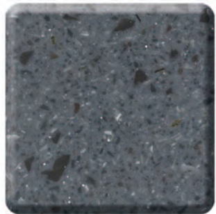
Ammonite
